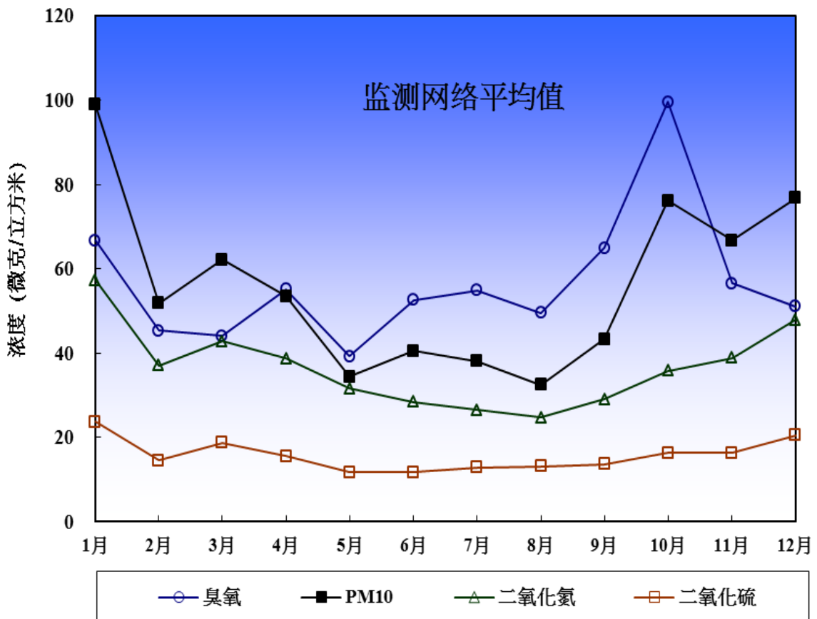
图 9: 监测网络污染物浓度平均值月际变化
